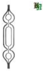
арт.691 210x1000мм, кв.12x12мм, вес 3,500кг Цена: 1400 руб.
