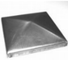
Заглушка, арт. 15.057 100x100x1мм Вес: 0.11 кг Цена: 34 руб.
