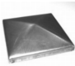
Заглушка, арт. 15.054 50x50x1мм Вес: 0.041 кг Цена: 15 руб.
