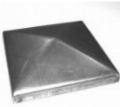
Заглушка, арт. 15.058 120x120x1мм Вес: 0.174 кг Цена: 55 руб.
