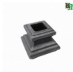
Вставка в балясину, арт. 1376.16 23x39мм, на кв.16x16мм Вес: 0.08 кг Цена: 32,50 руб.
