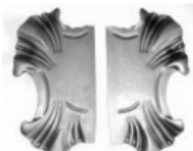
Накладка, арт. 4399-00 285x155x2мм Вес: 1.07 кг Цена (за пару): 340 руб.
