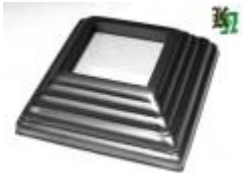
арт.13.319.01 80x80x1 кв. 30x30 вес 0,066 кг. Цена: *** руб.
